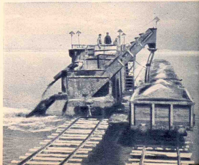
Мощный солесос на Таволжанском соляном промысле (Казахская ССР).
